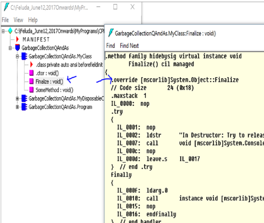
Figure 29-4. IL code
