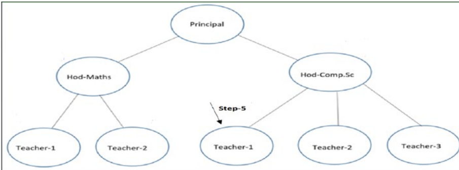
Figure 13-9. Step 5
